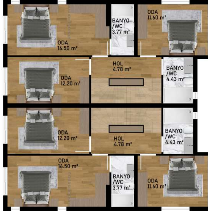
1. KAT PLANI
